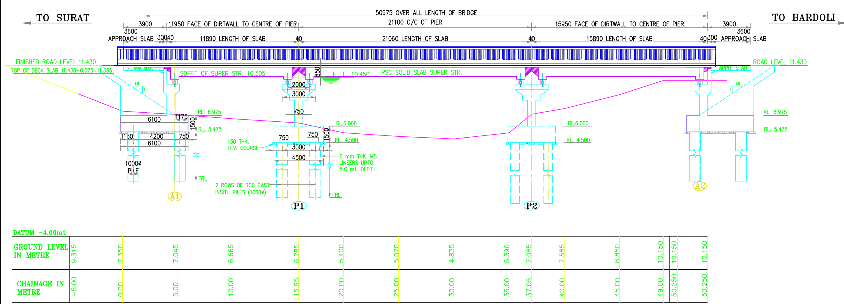
LONGITUDINAL ELEVATION AT A-A SCALE: 1:200
